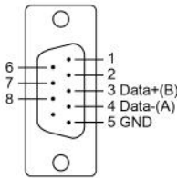
RS-485-2w
