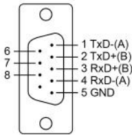
RS-422/RS-485-4w
